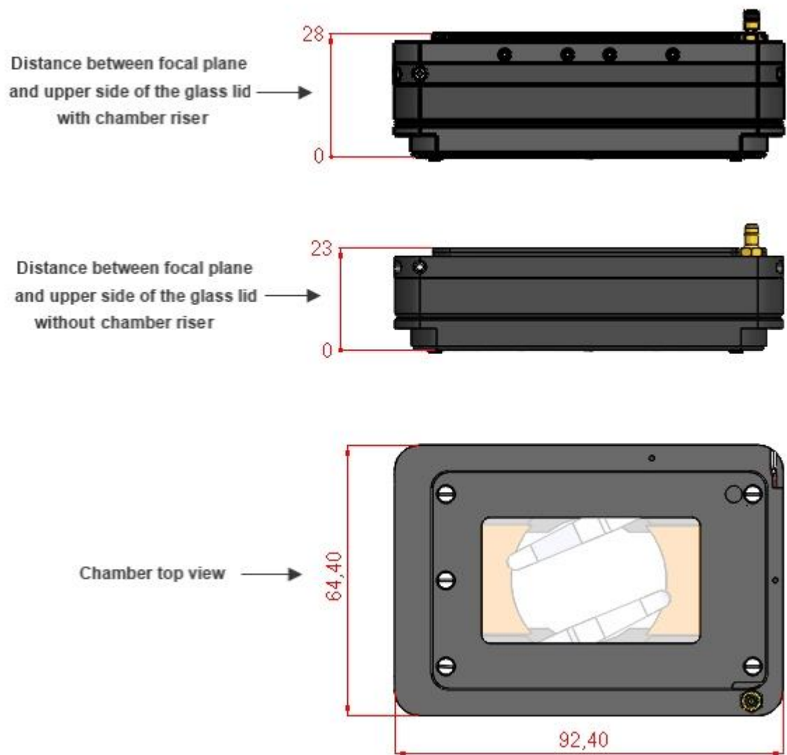
H301-PI-P-736-ZR1S/ZR2S - Dimensions
